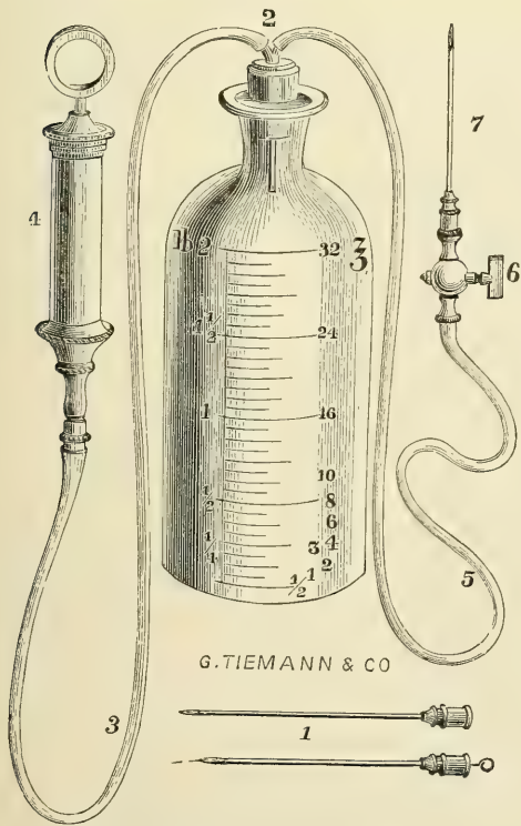
FIG. 576.—Tiemann & Co.'s aspirator.
